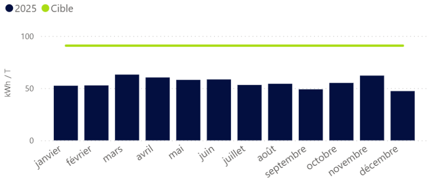
Evolution de la Consommation Elec (kWh) / Tonnes Triées
