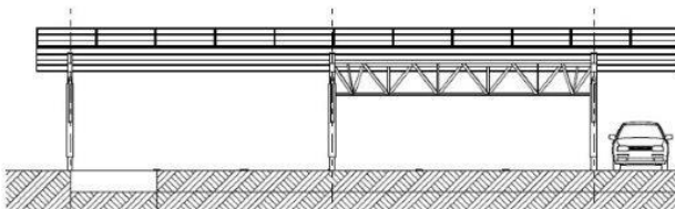
Plan de coupe des ombrières photovoltaïques
